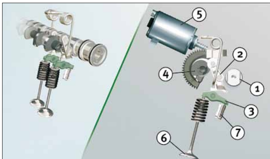
Снимка 1: Общ преглед на системата BMW Valvetronic/Подробен изглед на компонентите на системата.
