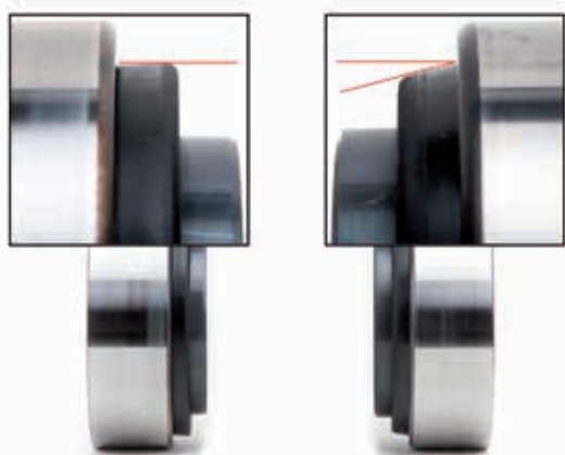
Снимка 1: Дизайнът на защитния капак за прах бе променен
